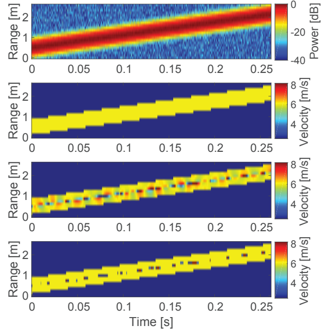
図1 上から順に信号強度 |s(t, r)|^2 、真の速度 v_0 、従来のテクスチャ法 v_{tex}(t, r) および提案法 v_{prop}(t, r) による推定速度
